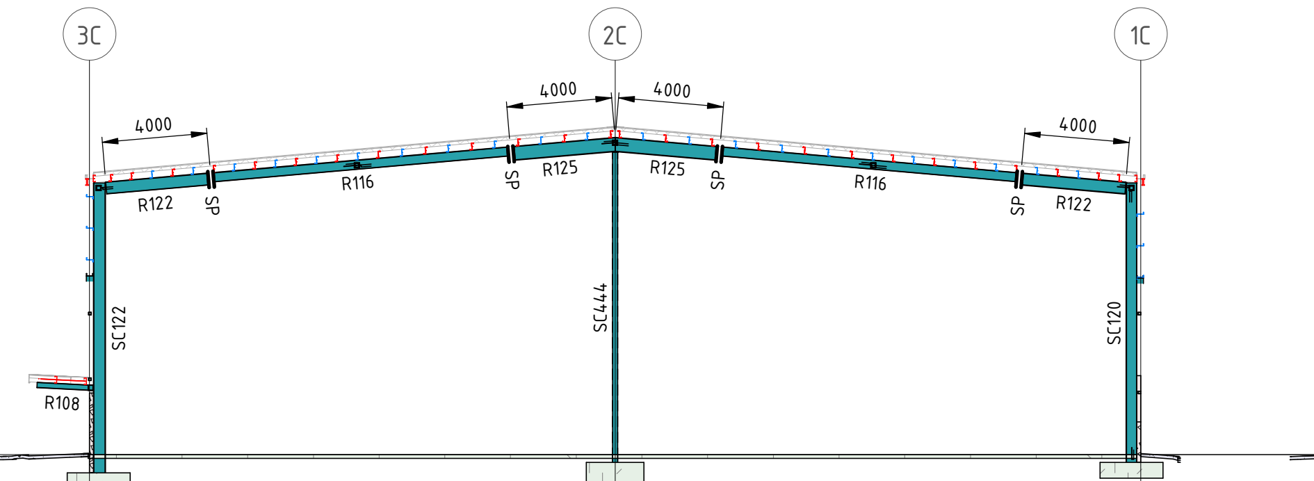
SECTION C9 SCALE 1 : 200
