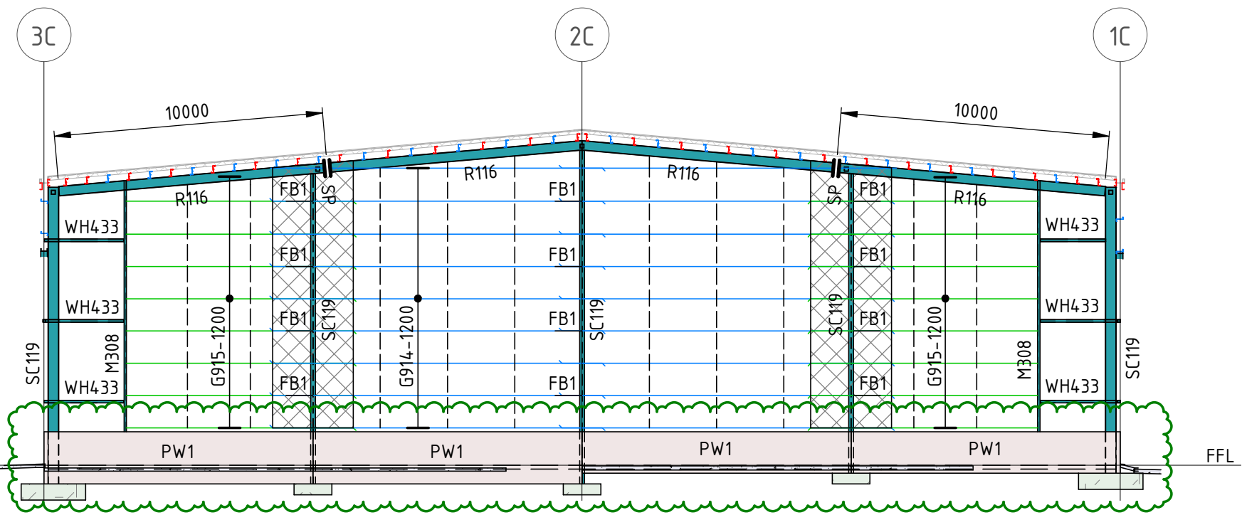
SECTION C10 SCALE 1 : 200
