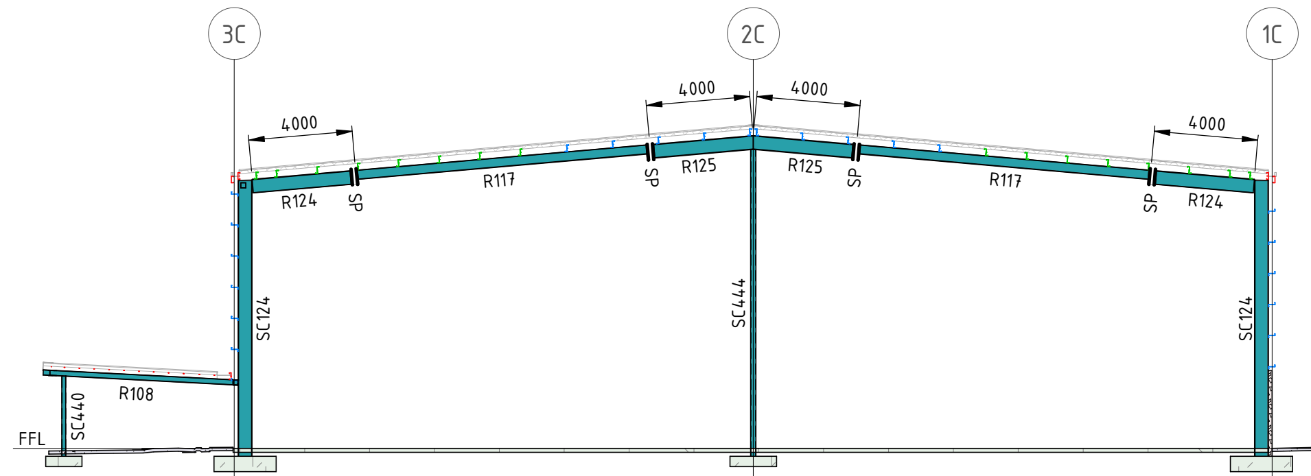
SECTION C4 SCALE 1 : 200
