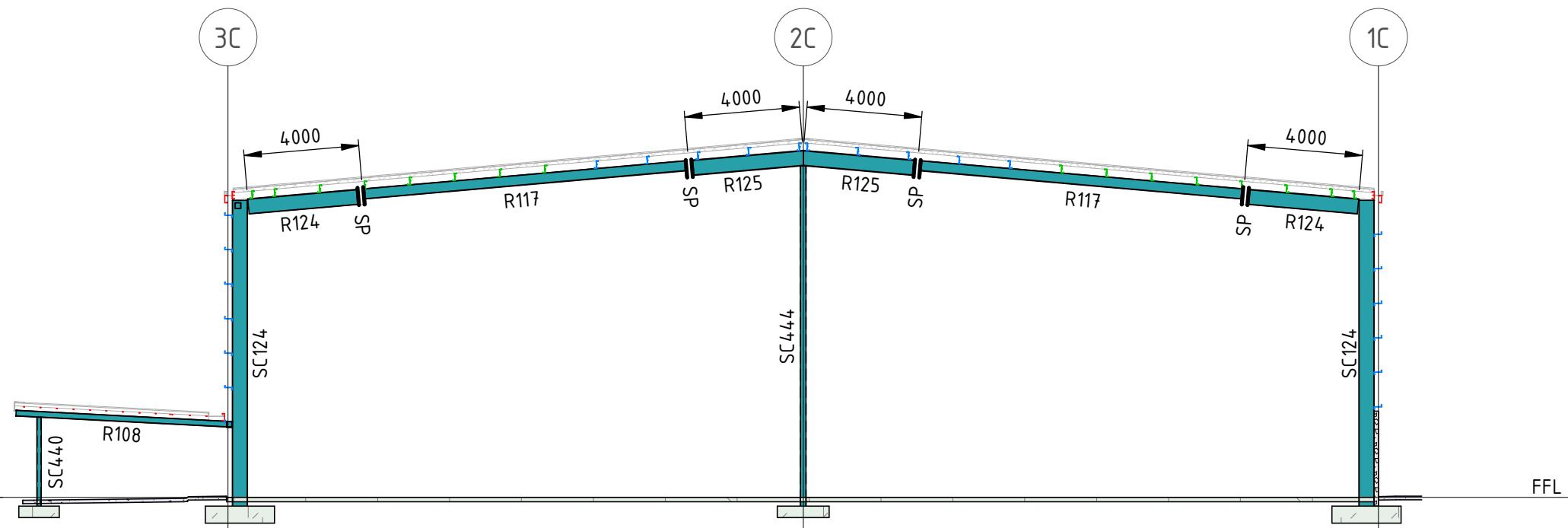
SECTION C5 SCALE 1 : 200
