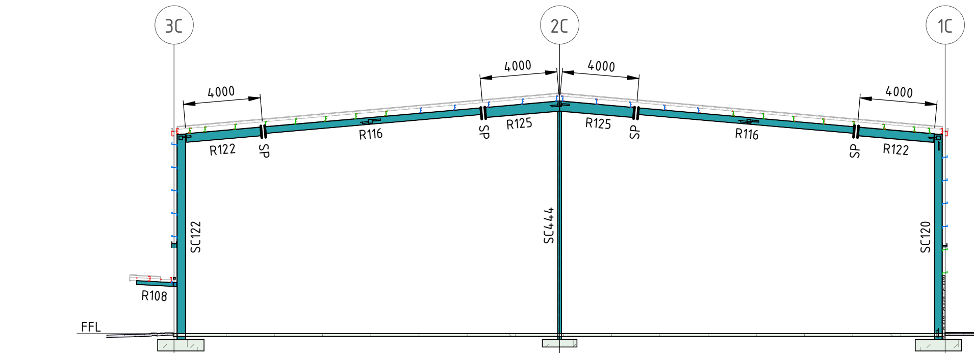
SECTION C8 SCALE 1 : 200
