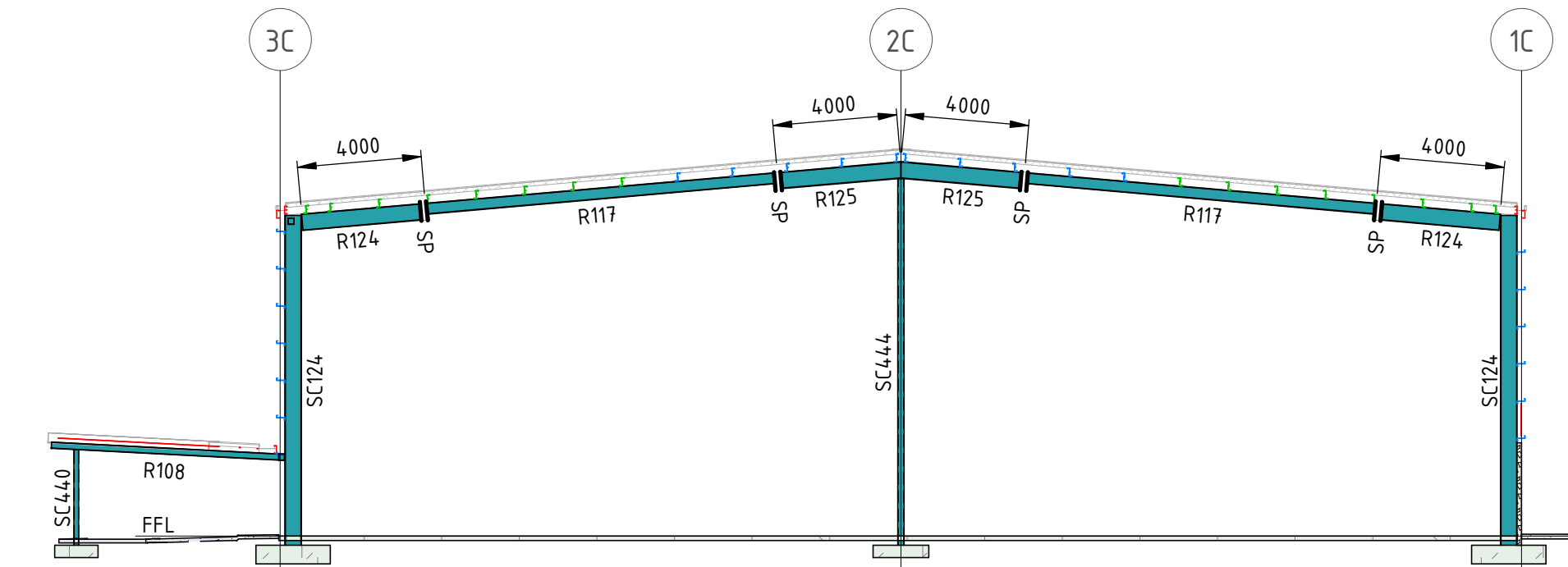
SECTION C6 SCALE 1 : 200
