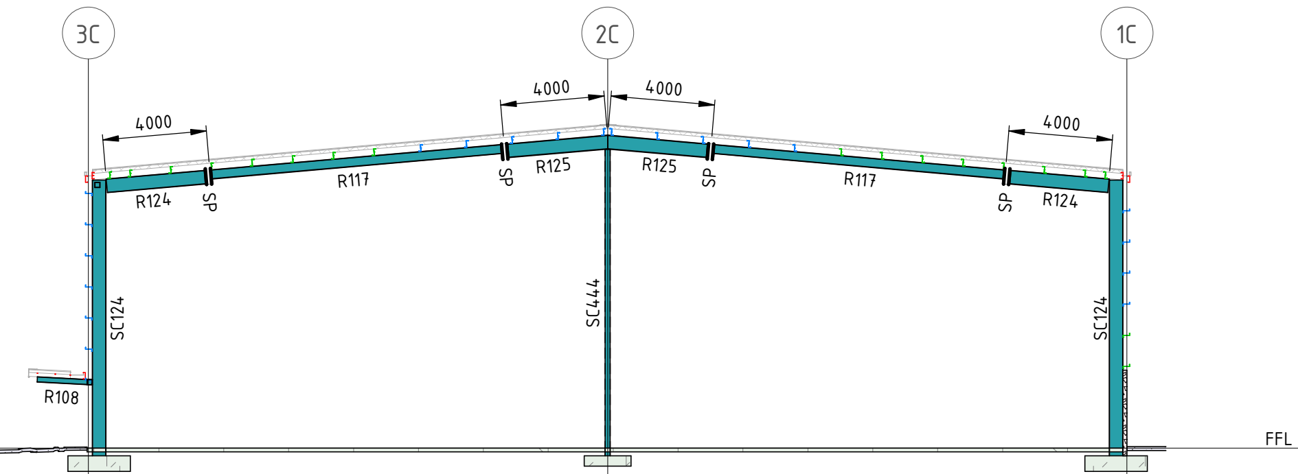
SECTION C7 SCALE 1 : 200
